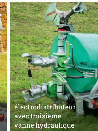
Électrodistributeur avec élément en T et couvercle
